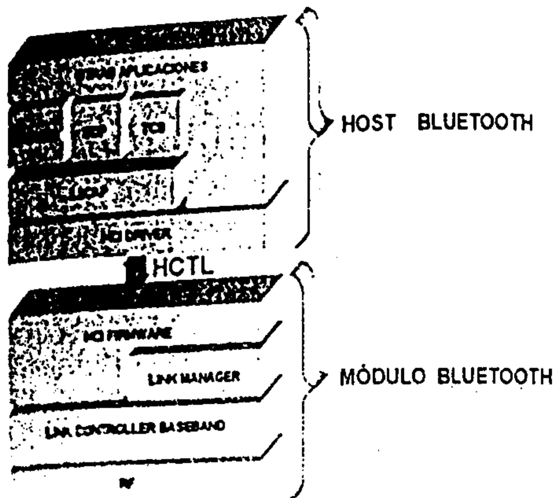
Figura 1. Arquitectura de protocolos de Bluetooth
